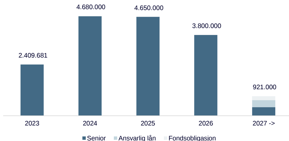
Figur 10 - Forfallstruktur verdipapirgjeld
